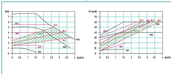
· ESPXX-7.5 III výkonová křivka
